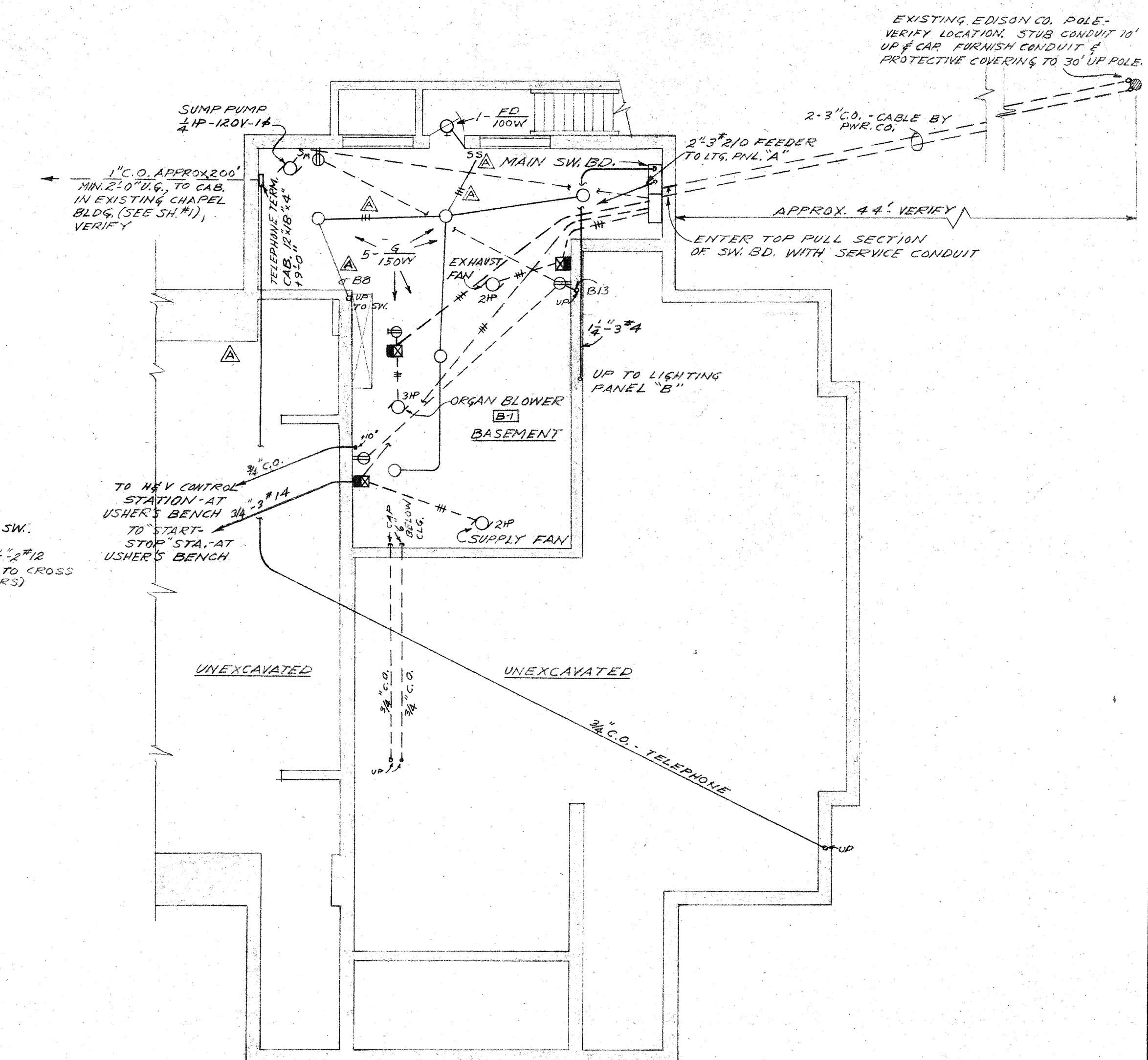
PLAN - BASEMENT SCALE: 1/8" = 1'-0"
